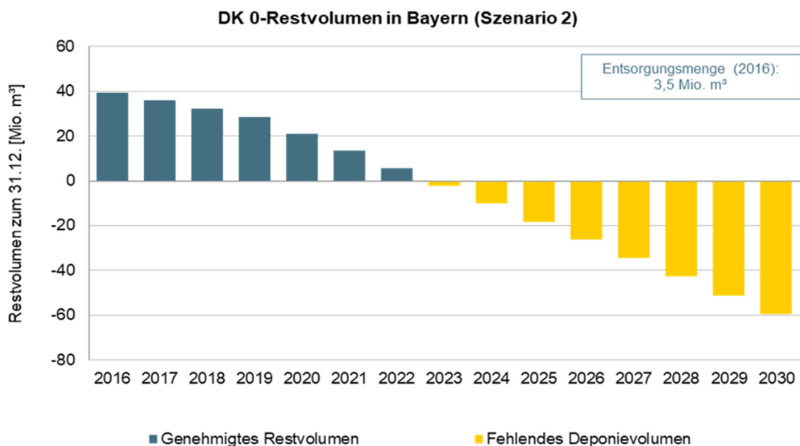
Abbildung 2 Entwicklung von Restvolumen und Deponiebedarf für DK 0-Deponien (Szenario 2 entspricht dem Inkrafttreten der Mantelverordnung)
