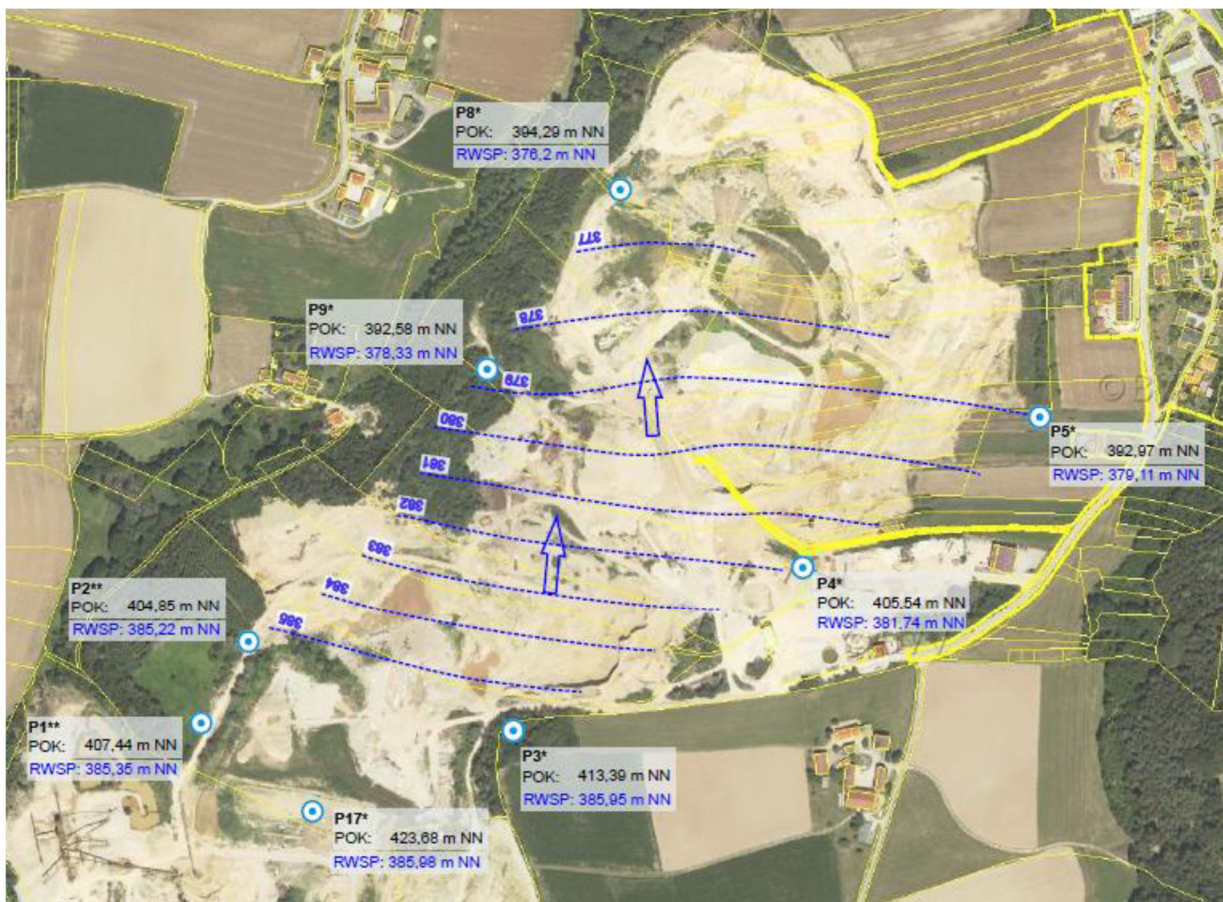
Abbildung 4 Lage der Grundwasserbeobachtungsstellen Zöls (Aufstandsfläche der geplanten Deponie mit Grundwassergleichen vom 06.12.2022)
