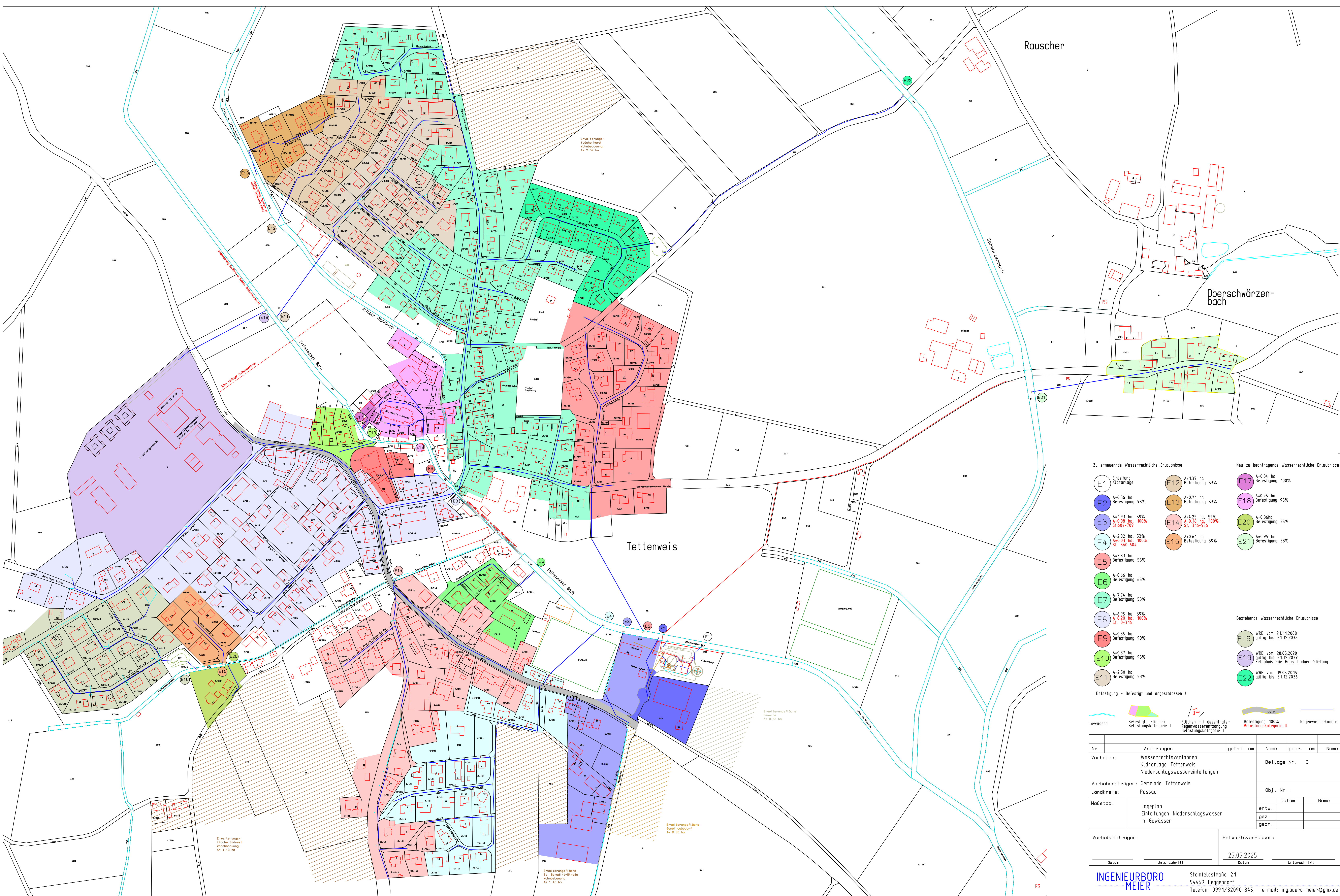
Lageplan Einzugsgebiete Niederschlagswasserkanalisation und Einleitungsstellen in die Gewässer
