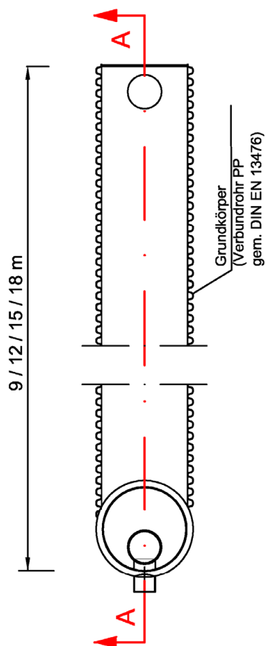
Schnitt C-C
