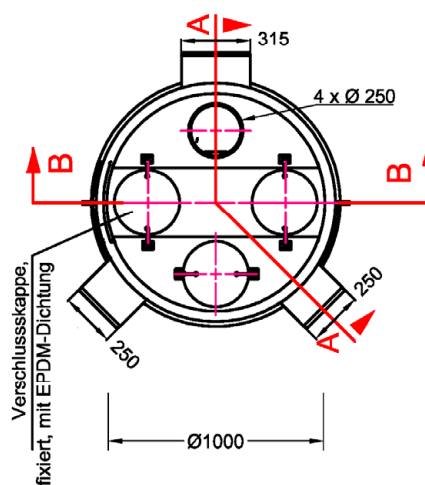
Draufsicht
