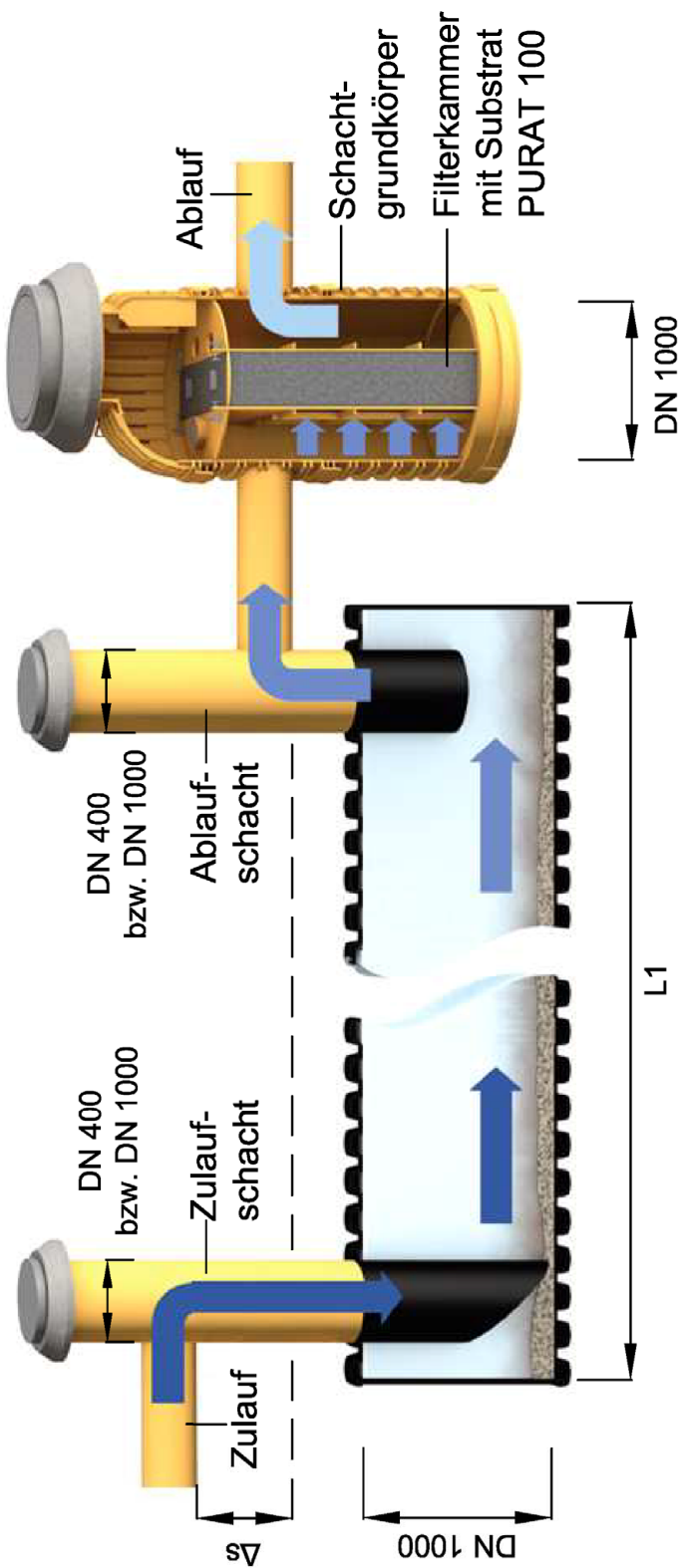
Filtrationsmodul
