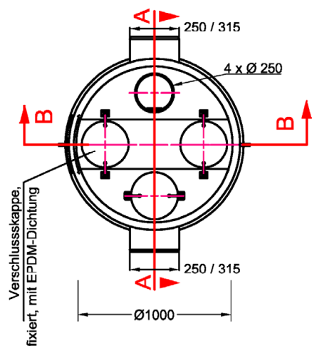
Draufsicht
