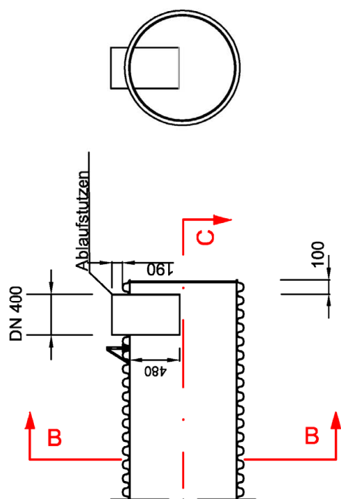
Schnitt B-B
