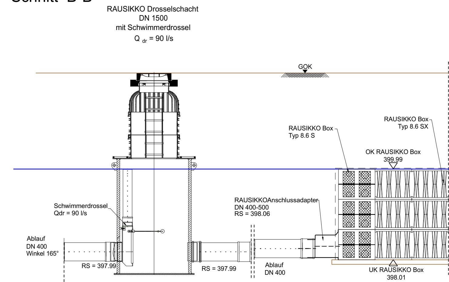
Schnitt B-B
