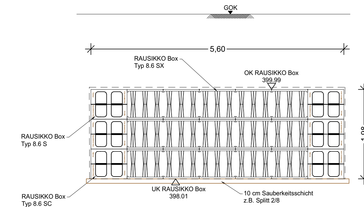
Schnitt C-C
