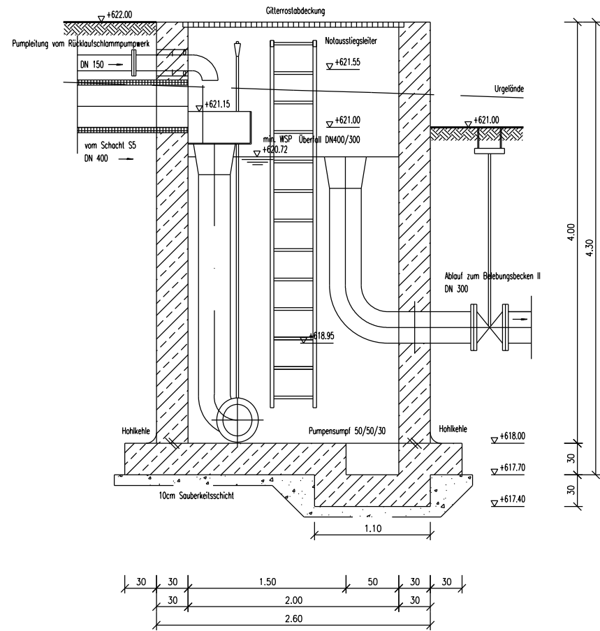
Schnitt A-A
