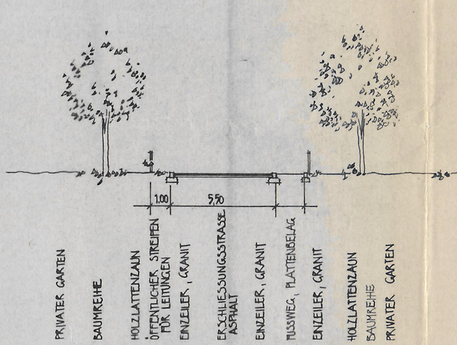
REGELSCHNITT 2 M 1:20
