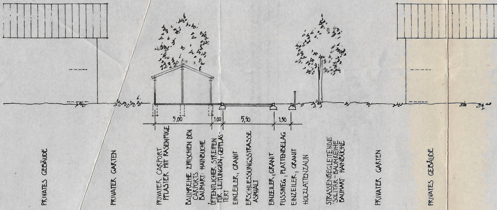
REGELSCHNITT 1 M 1:20
