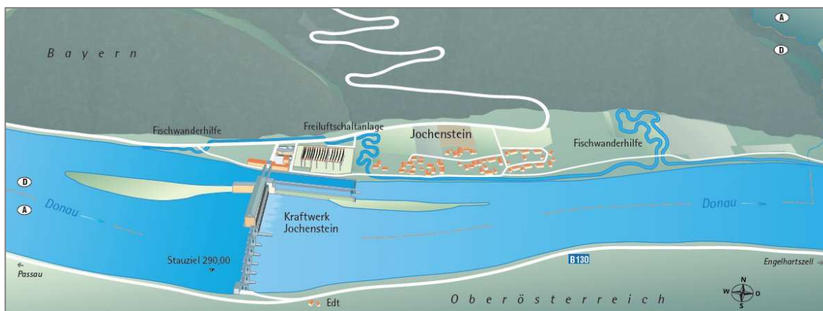
Bild 1: Projektübersicht Organismenwanderhilfe Kraftwerk Jochenstein
