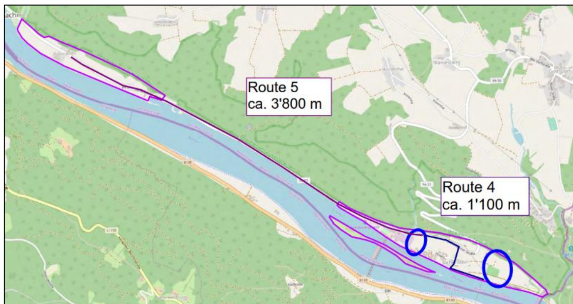
Abbildung 1: Transportabschnitte OWH
