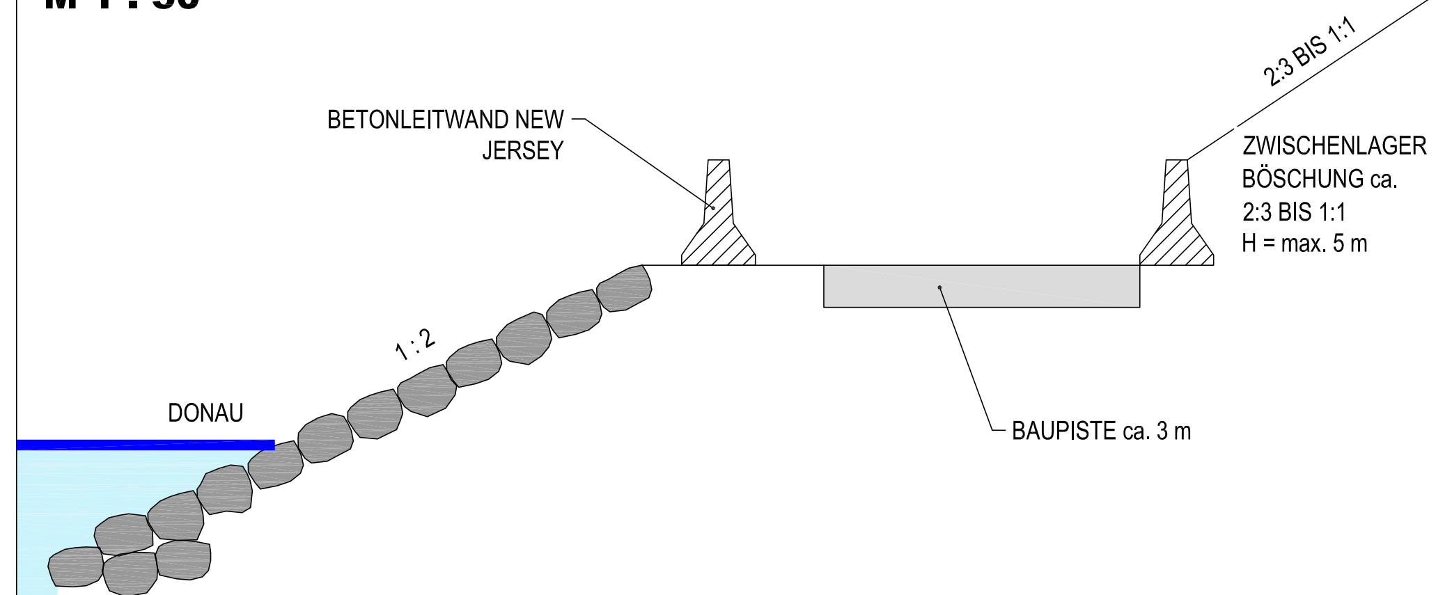
SCHNITT 1-1 BEREICH DONAU M 1 : 50
