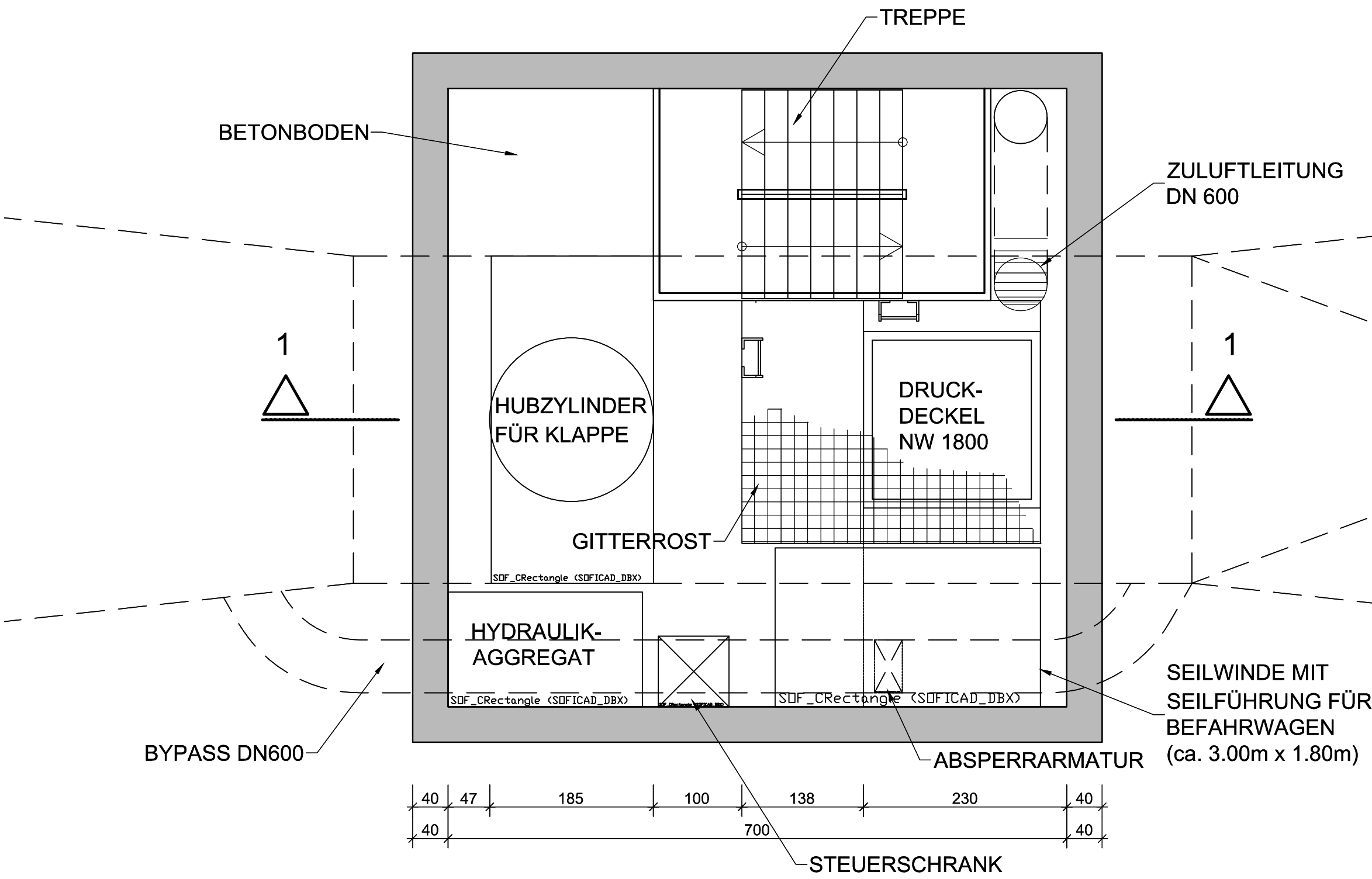
SCHNITT 3-3 M 1 : 50
