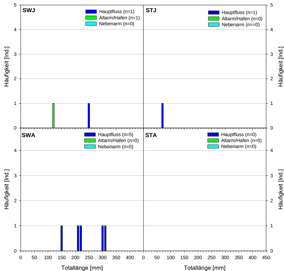
Abbildung 84: Populationsaufbau des Frauennerflings in den beiden Stauräumen 2019 (alle Methoden).
