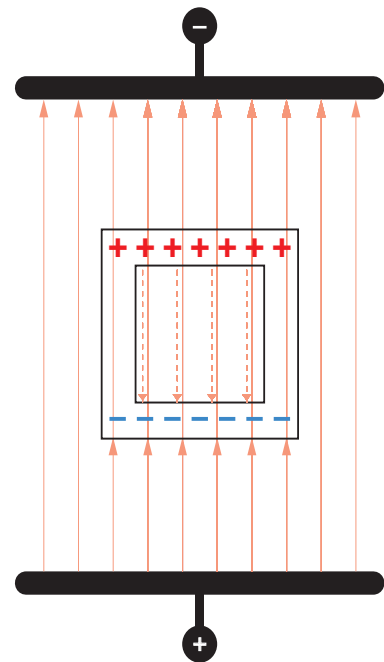
Abb. 3: Ein externes Feld führt bei guten Leitern zu einer Ladungsverteilung. Dadurch wird im Innern ein Gegenfeld erzeugt (im Bild gestrichelt dargestellt). In der Folge neutralisieren sich die Felder.
