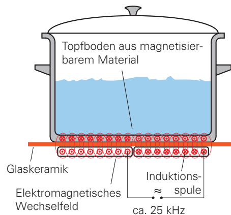
Abb. 41: Funktionsweise eines Induktionsherdes (schematisch).
