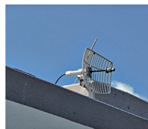
Abb. 70: WLAN-Richtfunksystem mit Gitter-Parabolantenne (5,8 GHz).
