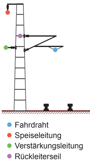
Abb. 29: Mögliche Leitungskonfiguration auf einem Fahrleitungsmasten der DB.
