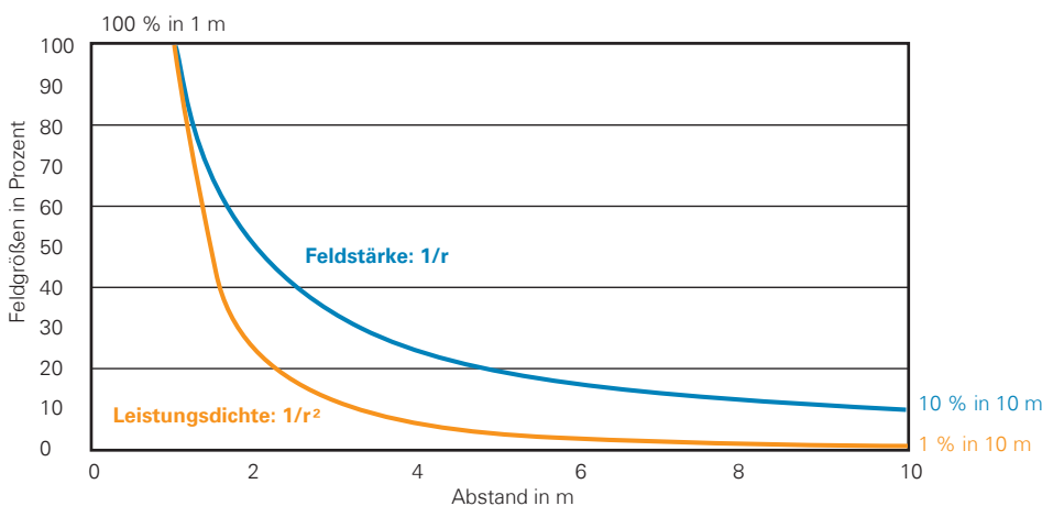
Abb. 46: Abnahme der Feldstärke und Leistungsdichte mit der Entfernung von der Quelle. Die Leistungsdichte nimmt bei zunehmendem Abstand von der Quelle umgekehrt proportional zum Quadrat des Abstandes ab ( 1/r^2 -Gesetz), die elektrische und die magnetische Feldstärke hingegen nur mit dem Abstand ( 1/r -Gesetz). Das bedeutet: Bei Verzehnfachung des Abstandes reduziert sich die Leistungsdichte auf ein Hundertstel des Ausgangswertes, die Feldstärke lediglich auf ein Zehntel.
